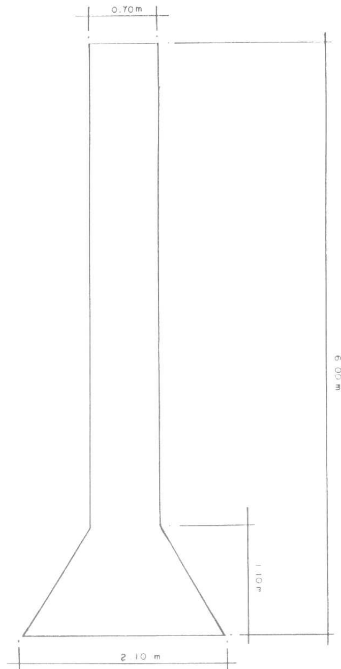
FIGURA 1 - Corte Vertical da Estrutura de um Poço Típico da Construção Civil Paulista.
